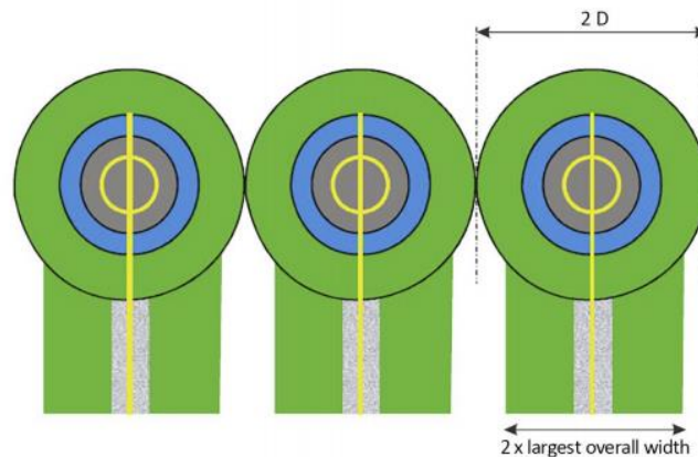
Figuur 16: Helikopter standplaats voor gelijktijdige operaties (EASA, 2019)
