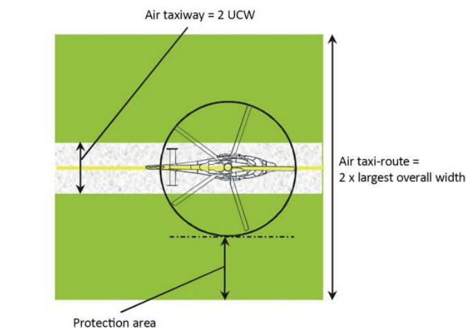
Figuur 15: Luchttaxibaan helikopter dimensie eisen (EASA, 2019)
