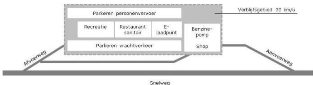
Figuur 22: Basisinrichting verzorgingsplaats (Rijkswaterstaat, 2019)
